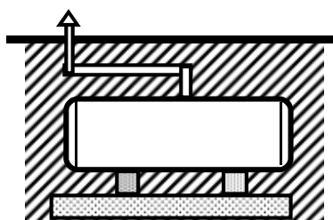
地下タンク貯蔵所 (69)
